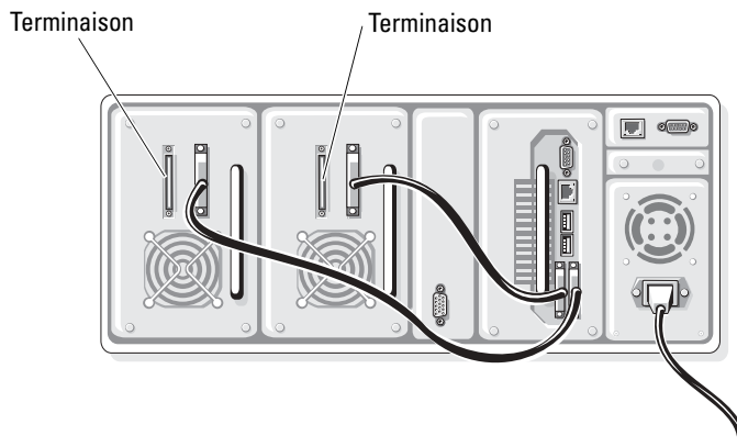
Figure 1-19. Bibliothèque de bandes comportant deux lecteurs
